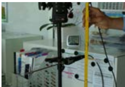
Abb. 10: Dritte Messung der Zugluft über dem Schreibtisch auf 1,1 m Höhe.
